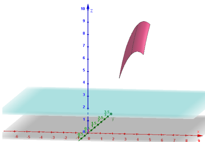
图 3.8 当 a = 7 时, 对 \forall x_1 \in [2, 4], \forall x_2 \in [1, 2] , 都有 f(x_1, x_2) \geq 2
