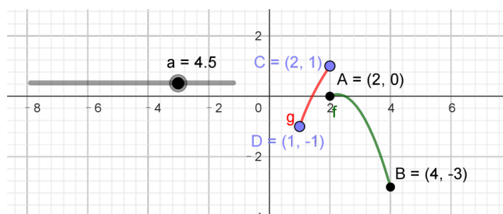
图 3.23 当 a = 4.5 时, 存在 f(x_1) 找不到 g(x_2) 比它小或与它相等
