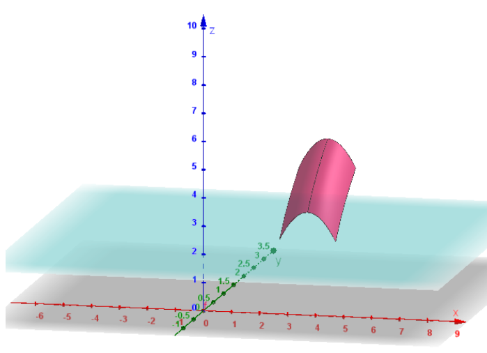
图 3.7 当 a = 6 时, 对 \forall x_1 \in [2, 4], \forall x_2 \in [1, 2] , 都有 f(x_1, x_2) \geq 2
