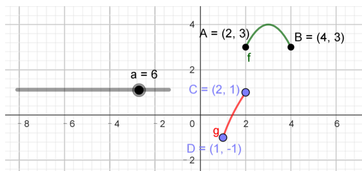
图 3.22 当 a = 6 时, 不存在 x_1 \in [2, 4], x_2 \in [1, 2] , 使得 f(x_1) = g(x_2) 成立
