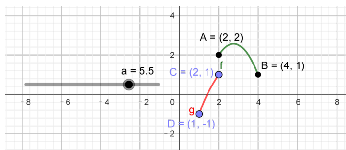
图 3.25 当 a = 5.5 时, 对任意的 f(x_1) 都有 g(x_2) 比它小或与它相等
