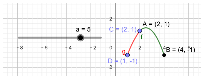
图 3.24 当 a = 5 时, 对任意的 f(x_1) 都有 g(x_2) 比它小或与它相等
